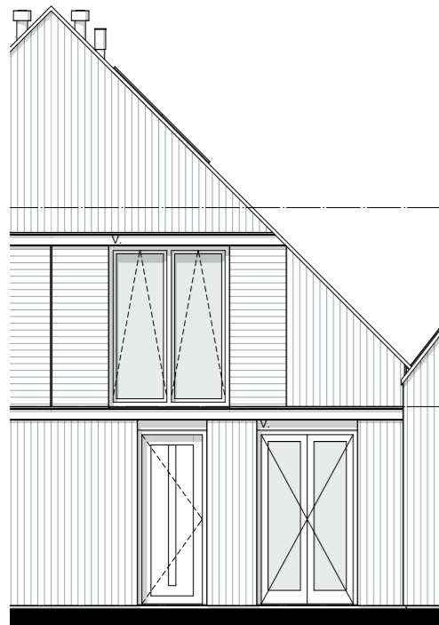
Voorgevel 1:100
