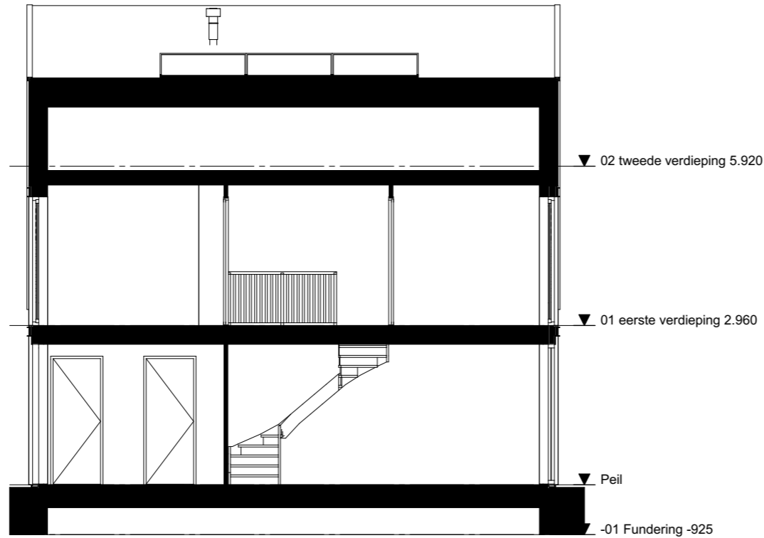
Doorsnede C-C 1:100
