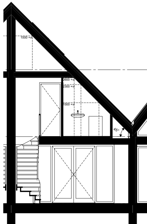
Doorsnede A-A 1:100
