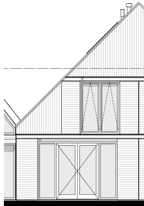
Achtergevel 1:100
