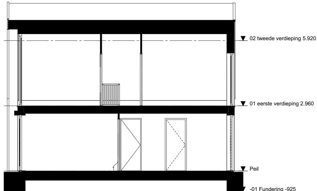
Doorsnede D-D 1:100
