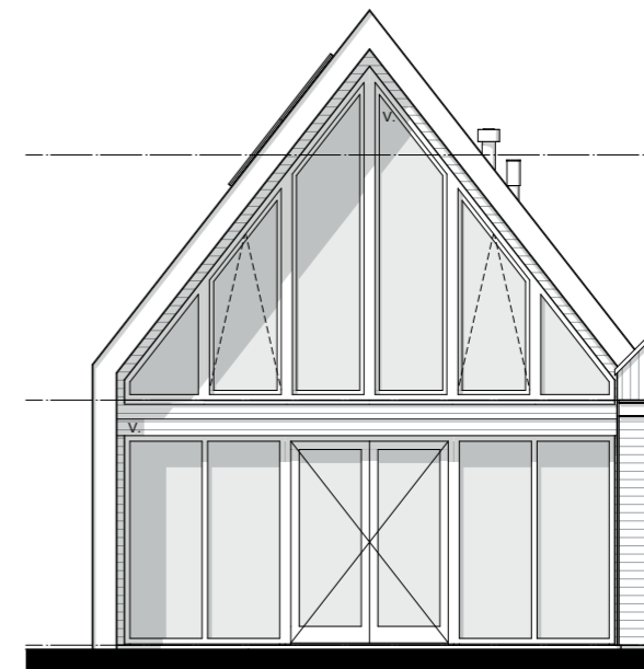
Achtergevel 1:100
