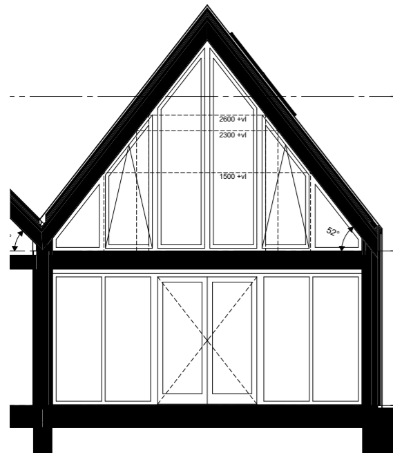
Doorsnede A-A 1:100
