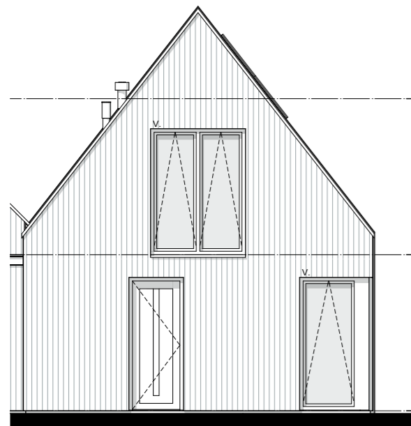
Voorgevel 1:100
